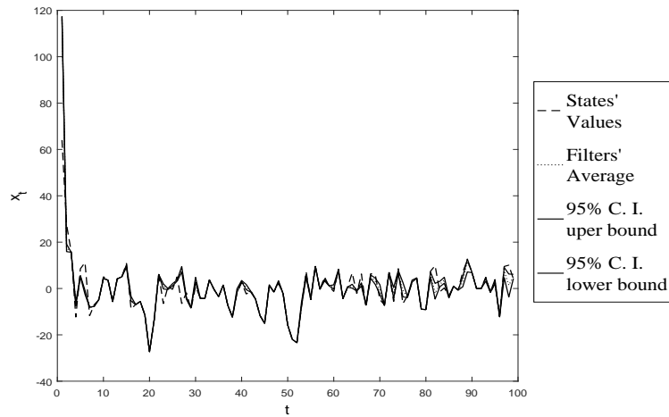
شکل ۳: میانگین عناصر بردار پالایش و فاصله اطمینان ۹۵٪، در ۵۰۰ بار شبیه‌سازی با مقادیر آغازین تصادفی در مدل (۶) با پارامترهای جدول ۲.
