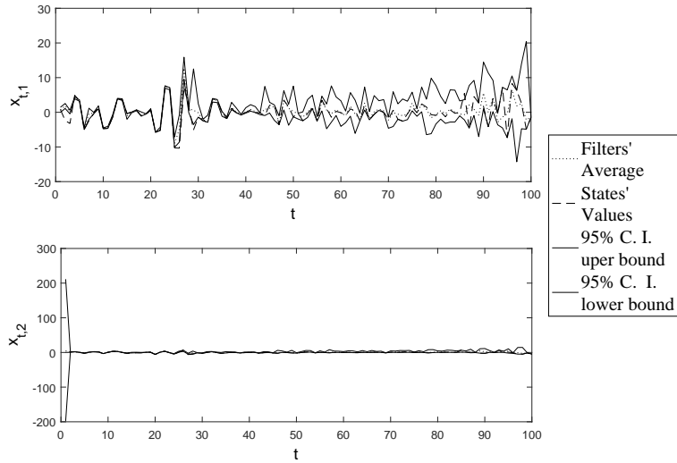
شکل ۱: میانگین عناصر بردار پالایش و فاصله اطمینان ۹۵٪، در 50^\circ بار شبیه‌سازی با مقادیر آغازین تصادفی در مدل (۶) با پارامترهای جدول ۱.
