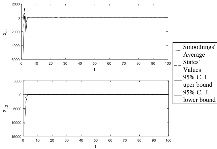
شکل ۲: میانگین عناصر بردار هموارسازی و فاصله اطمینان ۹۵٪، در 50^\circ بار شبیه‌سازی با مقادیر آغازین تصادفی در مدل (۶) با پارامترهای جدول ۱.
