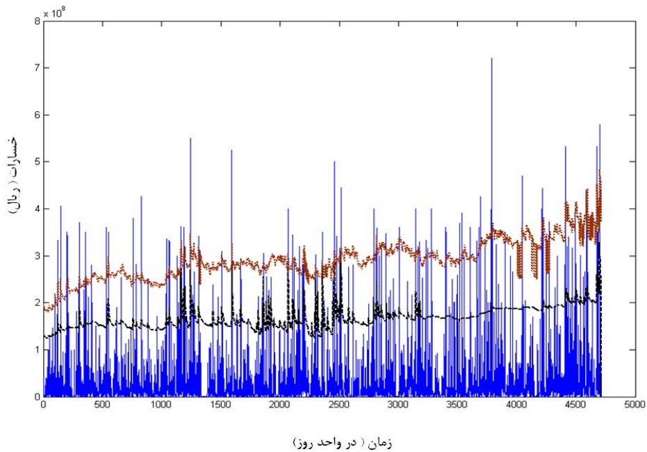
شکل ۶: خسارت‌های روزانه (خط)، برآورد مقدار در معرض خطر با استفاده از مدل‌های GARCH(1,1) (نقطه چین) و GARCH(1,1) (خط چین).
