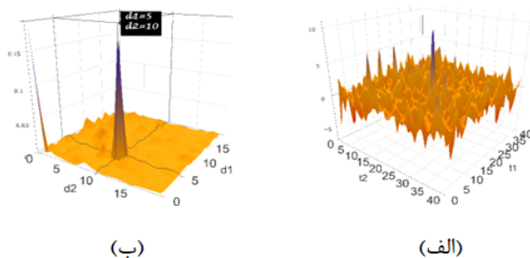
شکل ۳. الف: شبیه‌سازی فرآیند فضایی رابطه (۵). ب: دوره‌نگار فضایی این مدل
