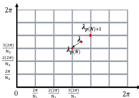
شکل ۱. نمایش فرکانس فوریه متناظر با \lambda
