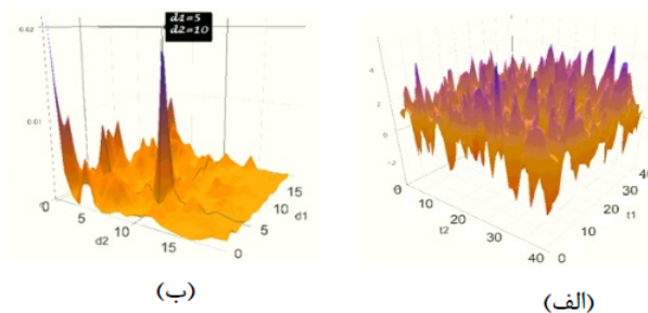
شکل ۳. الف: شبیه‌سازی فرآیند فضایی رابطه (۶). ب: دوره‌نگار فضایی این مدل.
