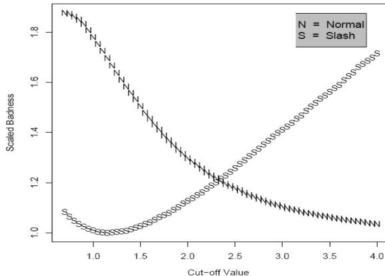
شکل ۲: نمودار مقادیر شبیه‌سازی شده b_{SC}^S(\lambda) و b_{SC}^G(\lambda) در ازای n = 5 و \underline{\lambda} = \{0/7, 0/75, \dots, 3/95, 4\}
